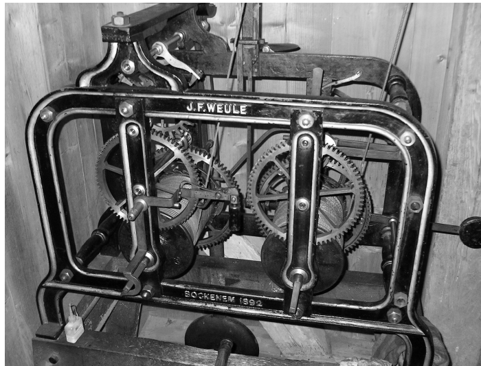
Abb. 12: Uhrwerk von 1892
